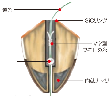
シモリ玉3部 松山(ビエル)断面図 松次郎ウキ止め糸を使用。V字になるよう結び事によりウキ内部でひっきり遊動固定を実現。PAT.186311
