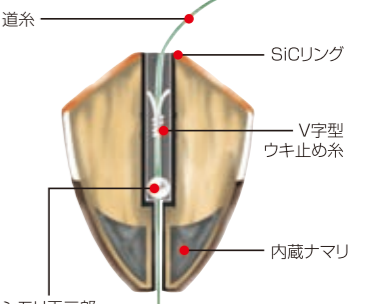
松山(ピエル)断面図 松次郎ウキ止め糸を使用。V字になるよう結び事によりウキ内部でひっきり遊動固定を実現。PAT.186311
